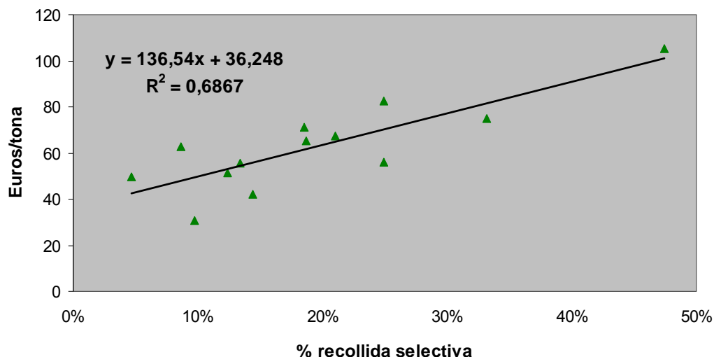
Gràfic 1. Relació entre els costos d'exploació de la recollida amb contenidors de superfície i els nivells assolits de recollida selectiva a diferents municipis representatius
